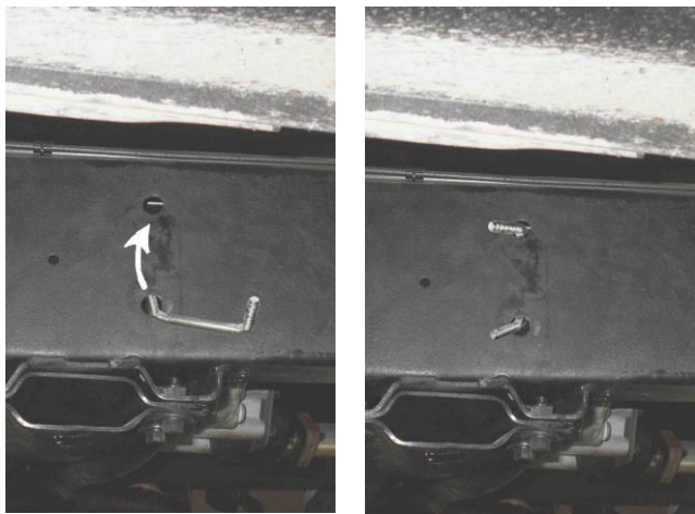
Рис. 4 Место крепления переднего кронштейна слева
