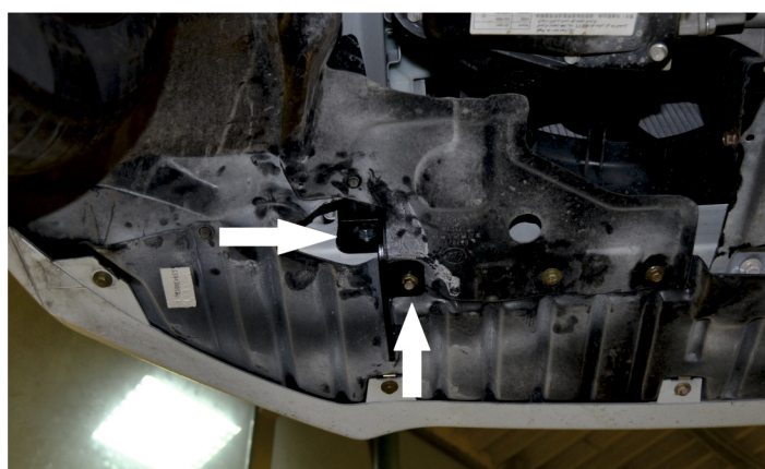
Рис. 1 - Установка кронштейнов
